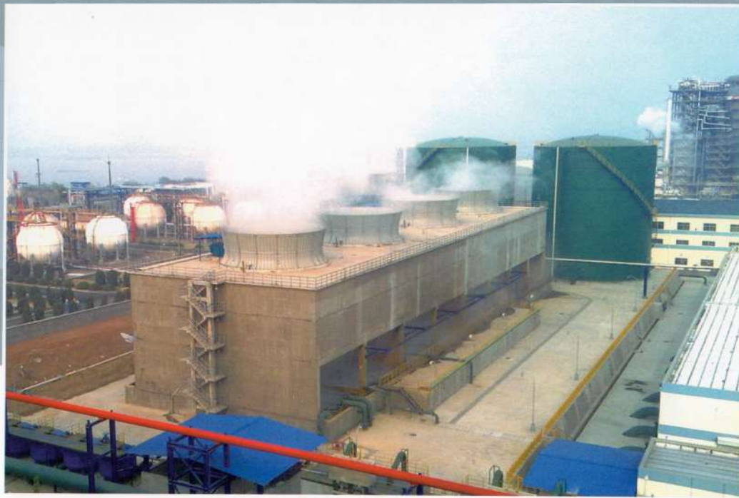
中石化金陵分公司 SINOPEC Jinling Company SHN-5500型冷却塔
