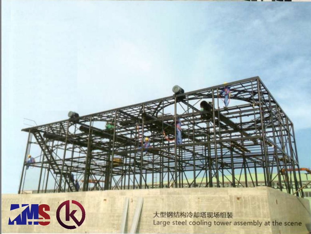
河南天方药业股份有限公司 Henan Tianfang Pharmaceutical Co., Ltd. NG-1500×3型钢网结构冷却塔
