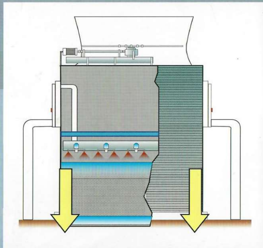
除雾节水型冷却塔示意图
